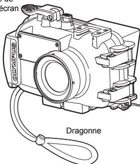
Corps du caisson
